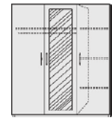
Drehtüreschrank 3-türig mittlere Tür mit Spiegel 1 Mittelwand 4 Einlegeböden 1 Kleiderstange
